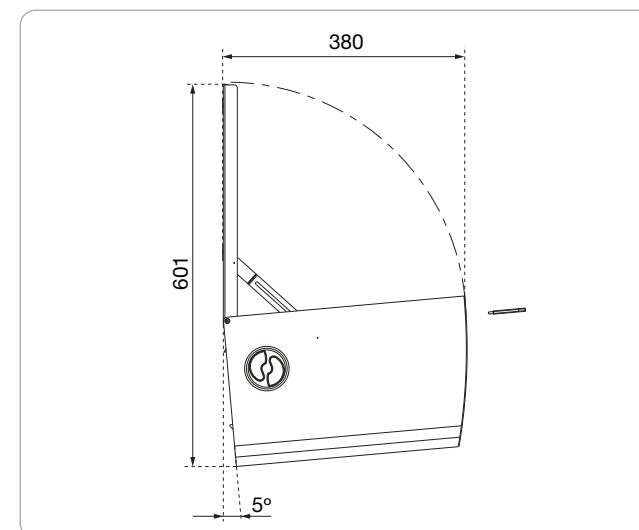
Seitenansicht.
